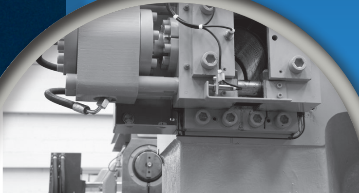
Säulenzieheinrichtung einer Druckgussmaschine der Bühler AG, Uzwil (Schweiz)
